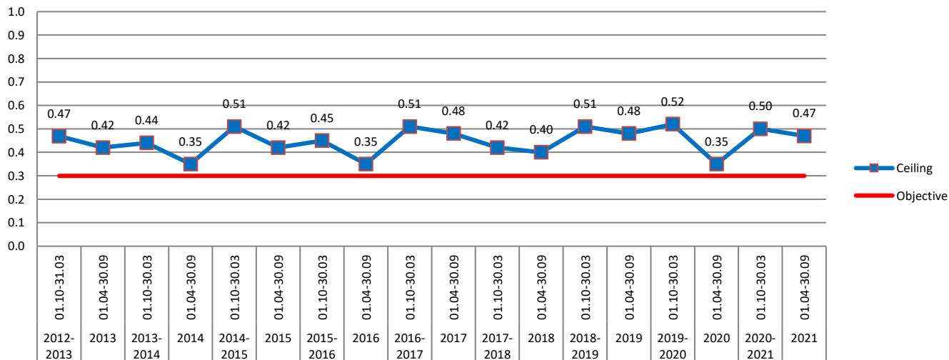
Plafond des nuages entre octobre 2012 et septembre 2021
